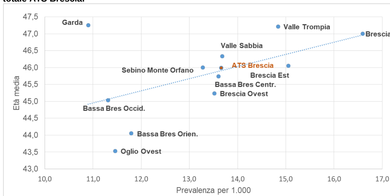
Figura 3. Grafico a dispersione dell'età media e prevalenza di demenza per distretto e totale ATS Brescia.
