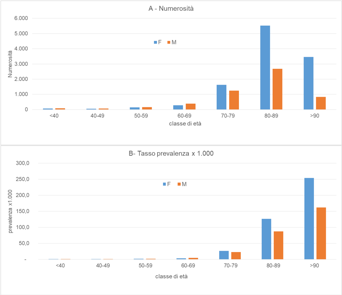
Figura 2. Numerosità (A) e prevalenza (B) della demenza per sesso e classe d'età in ATS Brescia. Anno 2024
