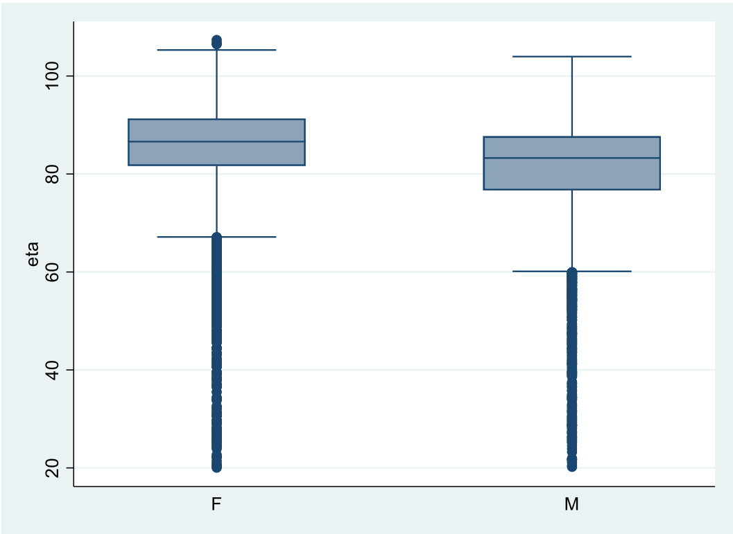
Figura 1. Box-plot della distribuzione dell'età degli assistiti con demenza, suddivisi tra maschi e femmine.
